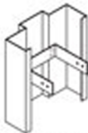
Wood stud anchor
